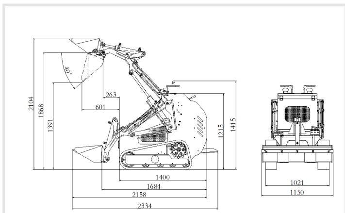
Dimensões principais
